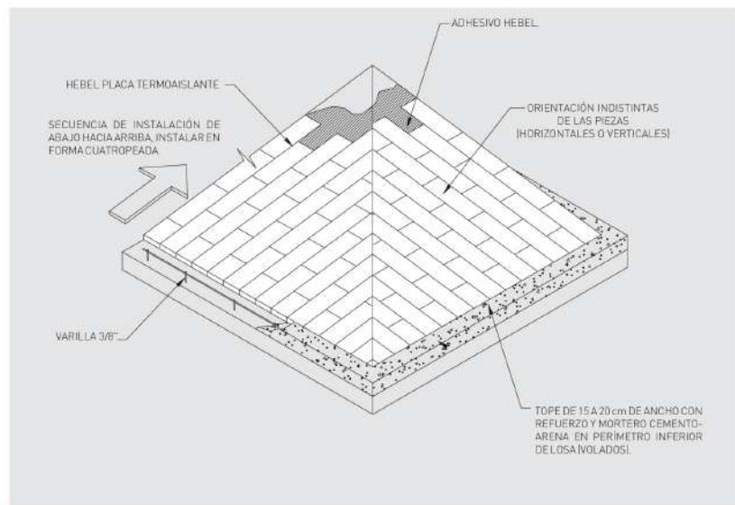
Fig.1: Hebel Placa termoaislante en losa inclinada.
